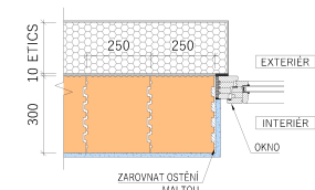
- VAZBA U OKENNÍHO OSTĚNÍ, 1. ŘADA ZDIVA
